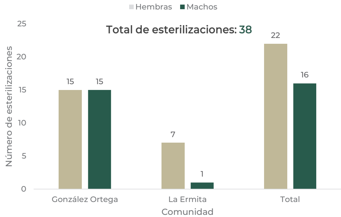
Gráfico 5. Número de esterilizaciones por comunidad, 2024.
