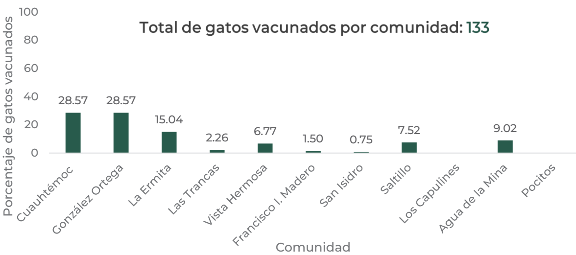
Gráfico 9. Porcentaje de gatos vacunados por comunidad, 2025.
