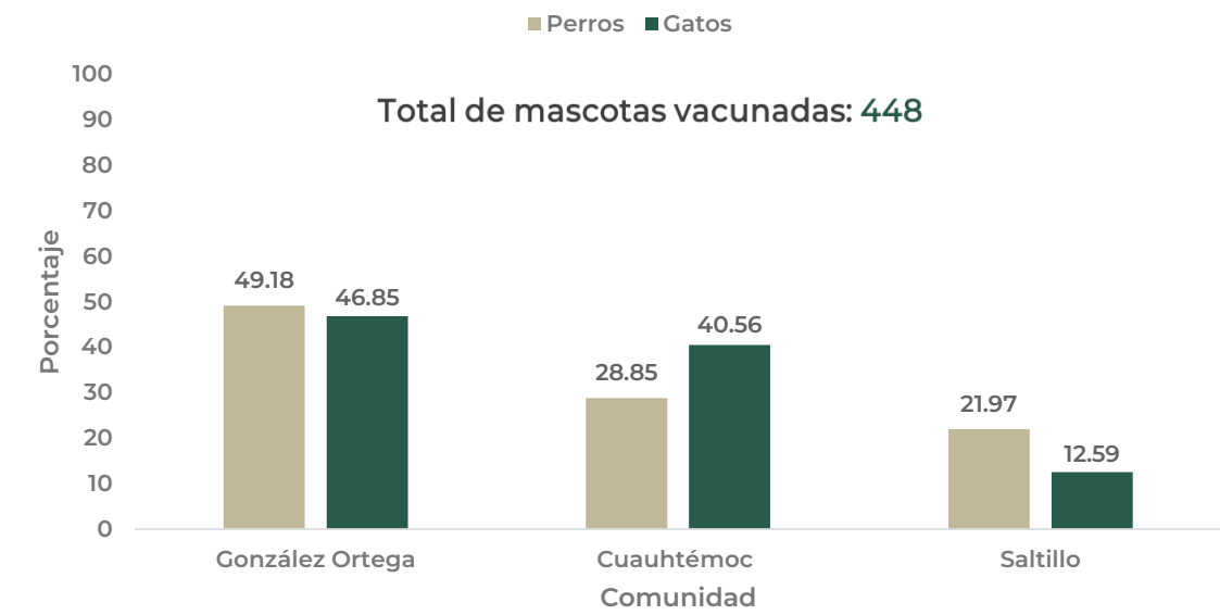
Gráfico 6. Porcentaje de perros y gatos vacunados por comunidad, 2024.
