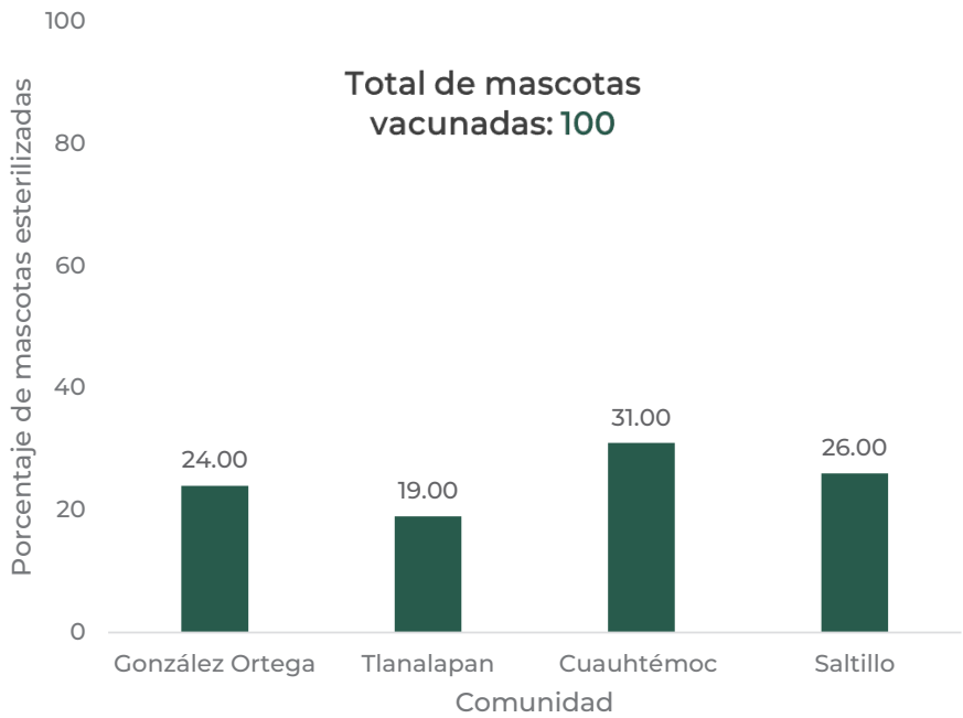
Gráfico 10. Porcentaje de mascotas esterilizadas por comunidad, 2025.
