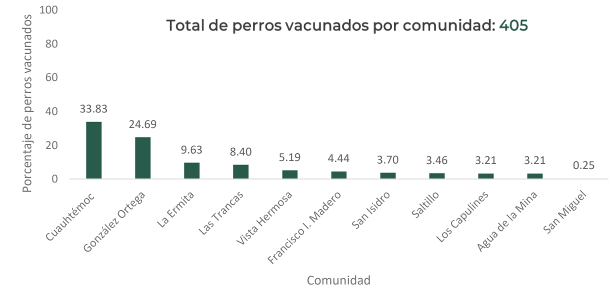
Gráfico 8. Porcentaje de perros vacunados por comunidad, 2025.
